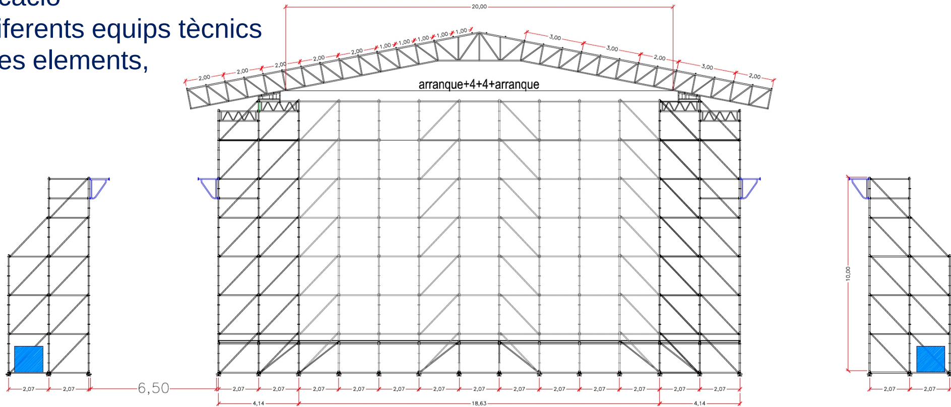
ALZADO FRONTAL
