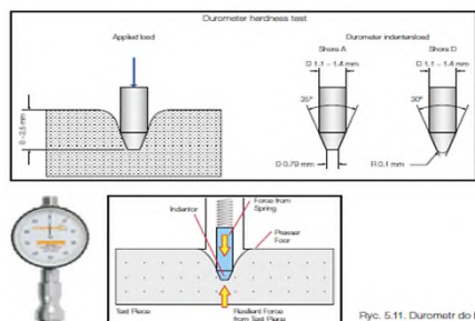
Foto: 5.11. Durometr de b Wöhle instruments, s.l.
