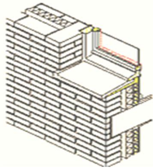
Fachadas convencionales de ladrillo
