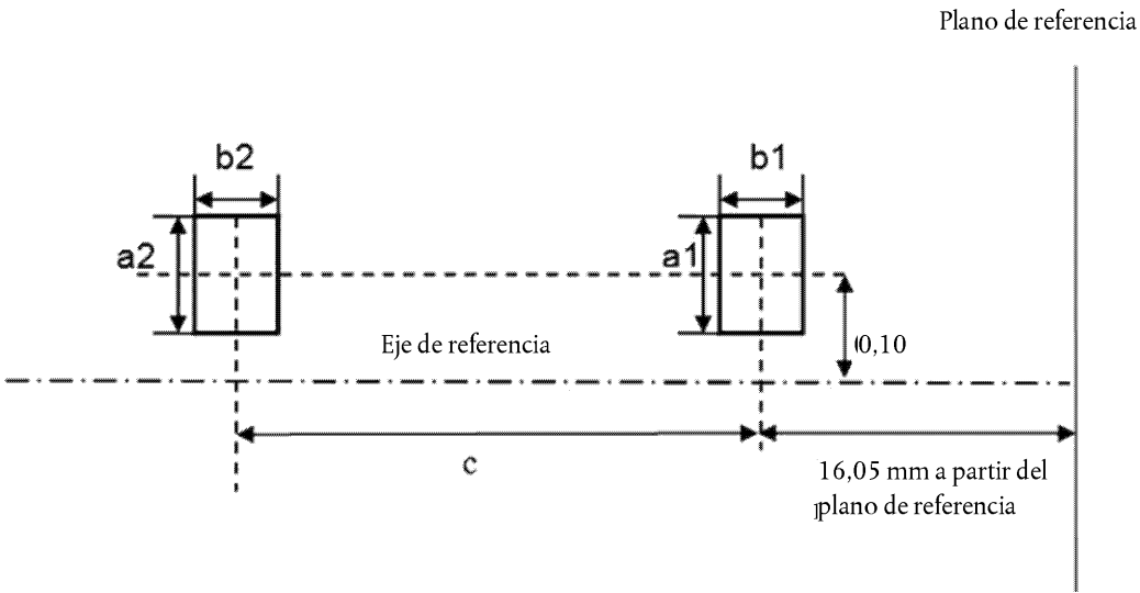
Vista lateral (esquemática):
